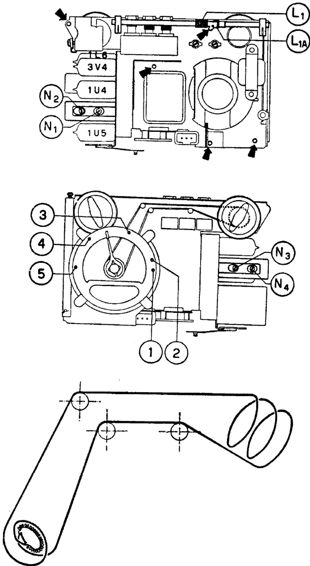
FARET - Portatile Voxson mod. 503 Dinghy - Posizione componenti e funicella comando scala.
